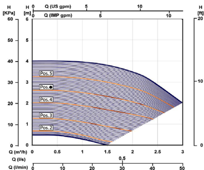
Fig. 4.4 – Caratteristiche elettropompa riscaldamento 3VS15-25/43
