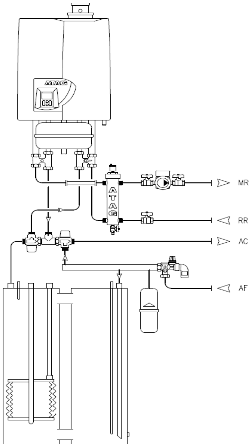
Fig. 12.2 – Componenti principali (boiler e circuito riscaldamento) A SOLAR modelli XXX/2
