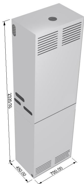
Fig. 6.1 – Dimensioni A SOLAR
