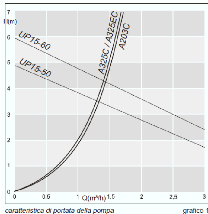
Fig. 7.1.C – caratteristica di portata generatori termici A SERIE
